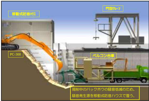
(施工設備配置状況 C G)
