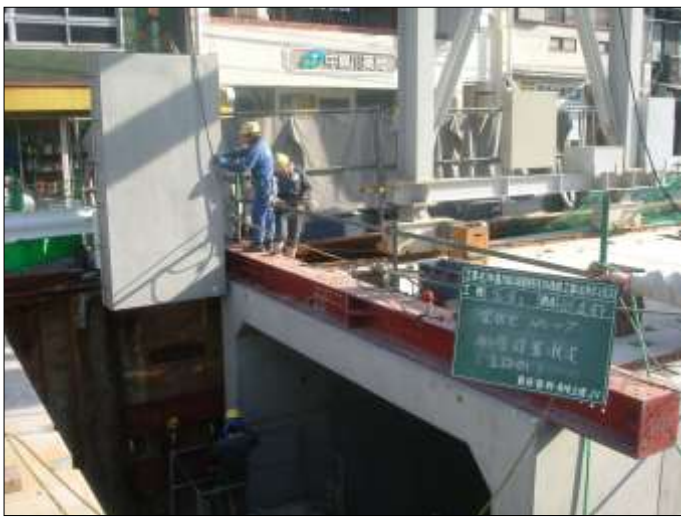
(側壁据付状況)
