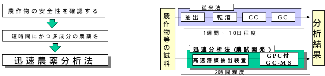
GPC+GC-MS
